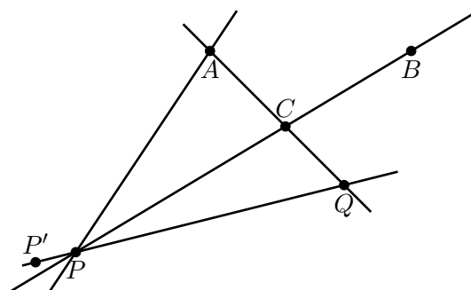
Abbildung 4.2: Situation aus Korollar 4.3
