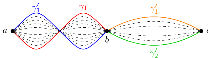
Abbildung 3.5: Situation aus Korollar 3.4
