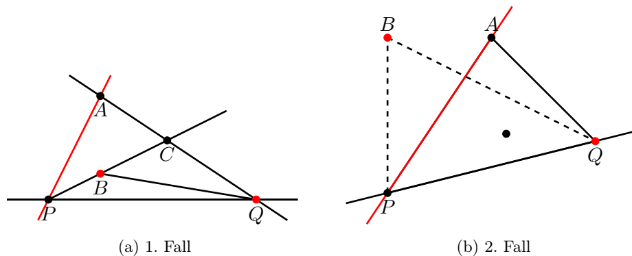
Abbildungung 4.4: Fallunterscheidung aus Korollar 4.4
