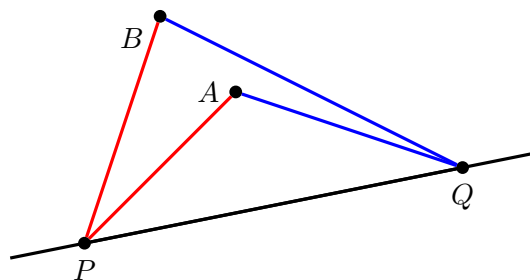
Abbildungung 4.3: Korollar 4.4: Die beiden roten und die beiden blauen Linien sind gleich lang. Intuitiv weiß man, dass daraus folgt, dass A = B gilt.
