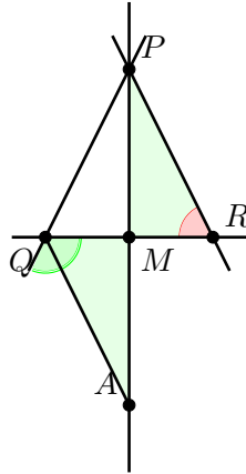
Abbildung 4.9: Situation aus Korollar 4.8
