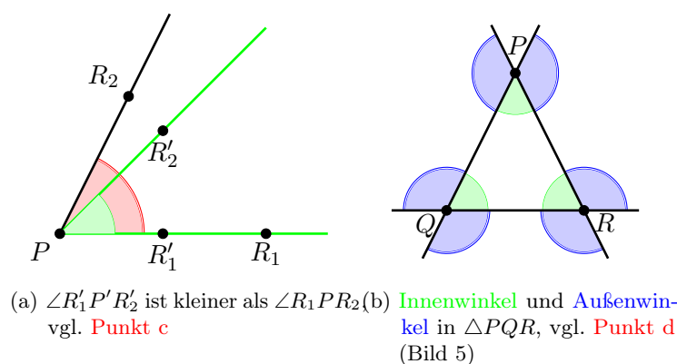
Abbildung 4.8: Situation aus Definition 56
