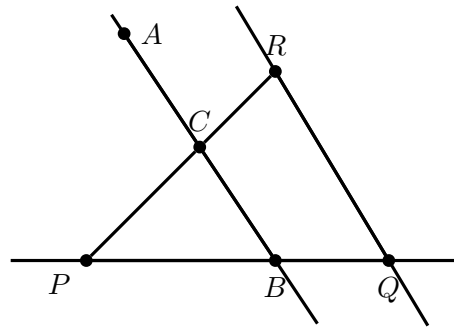
Abbildung 4.5: P, Q, R sind Fixpunkte, B \in \overline{PQ} \setminus \{P, Q\} , A \notin PQ \cup PR \cup QR
