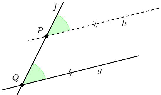
Abbildung 4.7: Situation aus Proposition 4.5
