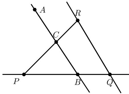
Abbildung 4.2: P, Q, R sind Fixpunkte, B \in \overline{PQ} \setminus \{P, Q\} , A \notin PQ \cup PR \cup QR
