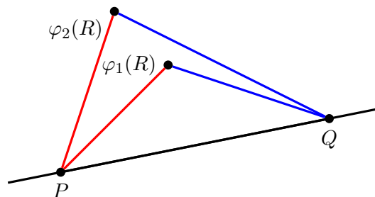
Abbildung 4.3: Die beiden roten und die beiden blauen Linien sind gleich lang. Intuitiv weiß man, dass daraus folgt, dass \varphi_1(R) = \varphi_2(R) gilt.
