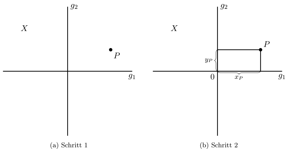
Abbildung 4.19: Beweis zu Satz 4.8
