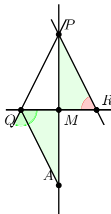
Abbildung 4.9: Situation aus Bemerkung 67
