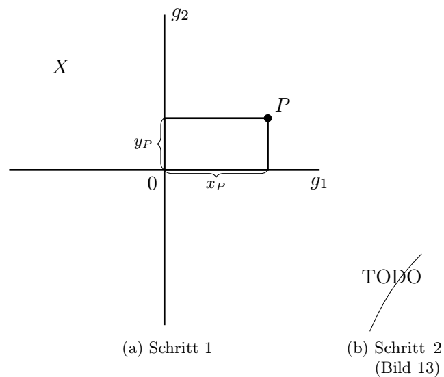
Abbildung 4.20: Beweis zu Satz 4.8
