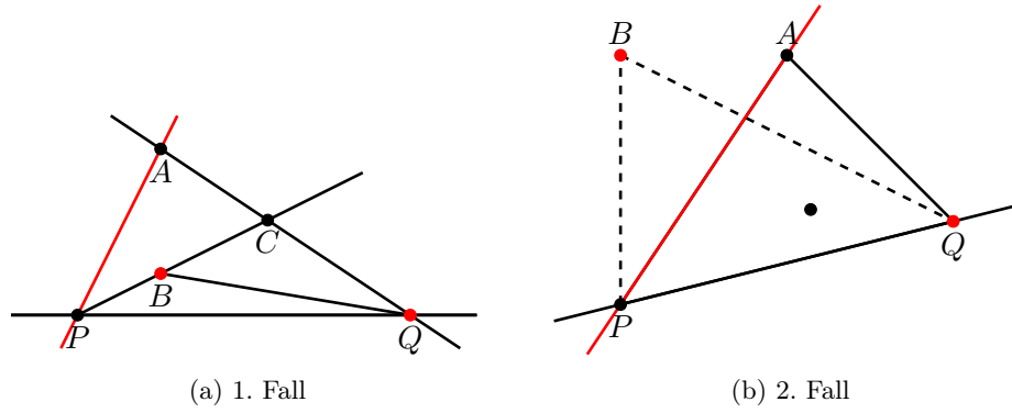
Abbildung 4.4: Fallunterscheidung aus Bemerkung 63
