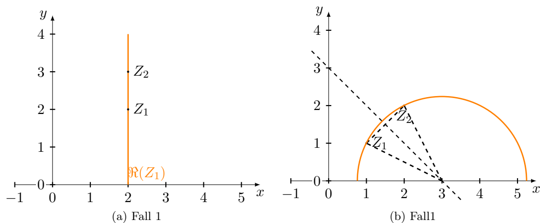
Abbildung 4.21: Zwei Punkte liegen in der hyperbolischen Geometrie immer auf genau einer Geraden
