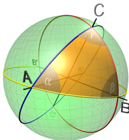
Abbildung 4.10: In der sphärischen Geometrie gibt es, im Gegensatz zur euklidischen Geometrie, Dreiecke mit drei 90°-Winkeln.
