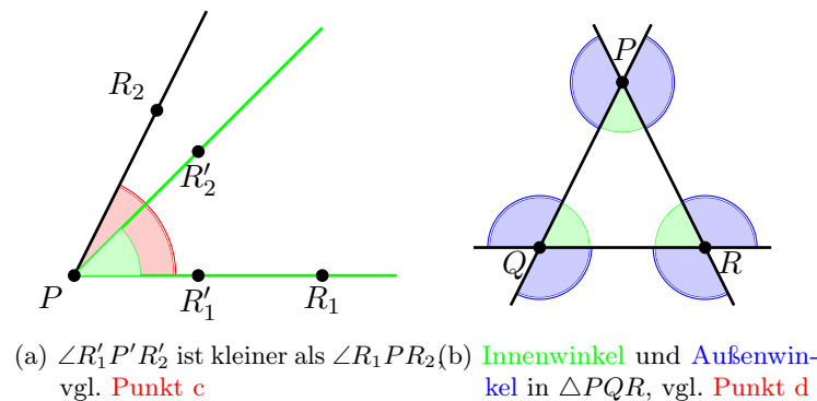
Abbildung 4.8: Situation aus Definition 57
