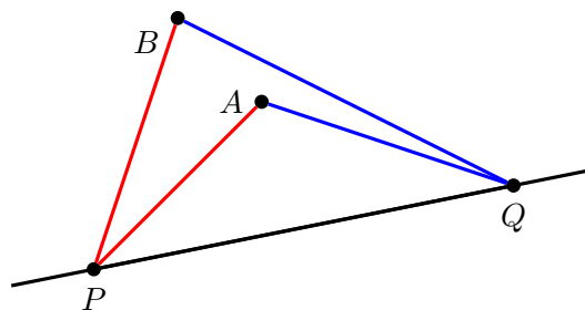
Abbildung 4.3: Korollar 4.4: Die beiden roten und die beiden blauen Linien sind gleich lang. Intuitiv weiß man, dass daraus folgt, dass A = B gilt.
