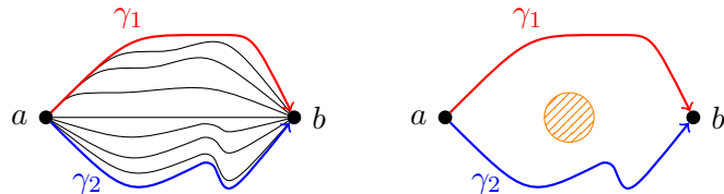
(a) \gamma_1 und \gamma_2 sind homotop, da man sie „zueinander verschieben“ kann. (b) \gamma_1 und \gamma_2 sind wegen dem Hindernis nicht homotop.
