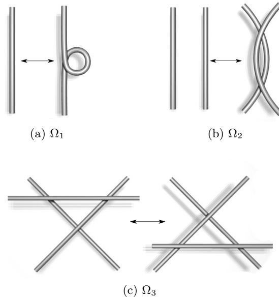
Abbildung 1.12: Reidemeister-Züge
