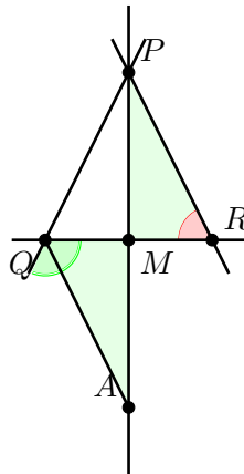
Abbildung 4.9: Situation aus Korollar 4.8
