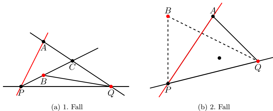
Abbildung 4.4: Fallunterscheidung aus Korollar 4.4
