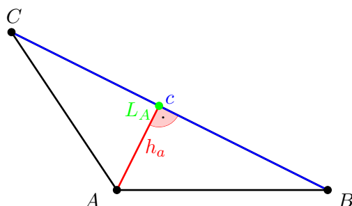
Abbildung 4.16: Flächenberechnung im Dreiecks
