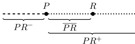
Abbildung 4.1: Halbgeraden
