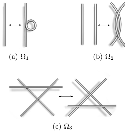
Abbildung 1.12: Reidemeister-Züge
