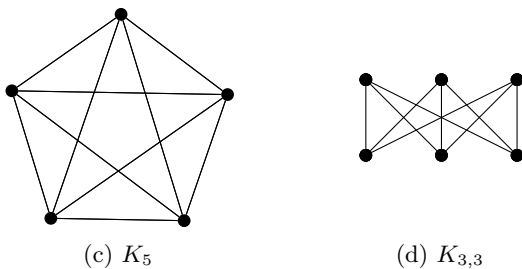
Abbildung 2.8: Beispiele für Graphen
