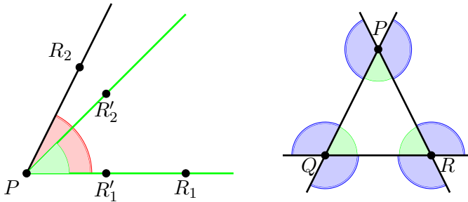
(a) \angle R'_1 P' R'_2 ist kleiner als \angle R_1 P R_2 (b) Innenwinkel und Außenwinkel in \triangle PQR , vgl. Definition 58.d
