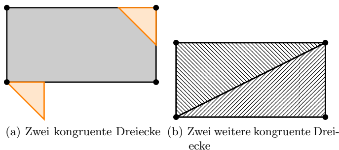
Abbildung 4.15: Flächengleichheit
