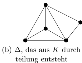
Abbildung 2.9: Beispiel für Bemerkung 36.
