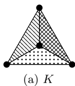
Abbildung 2.9: Beispiel für Bemerkung 36.
