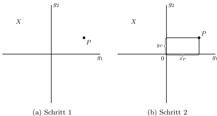
Abbildung 4.19: Beweis zu Satz 4.8
