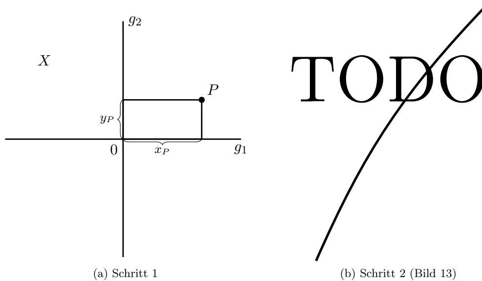
Abbildung 4.19: Beweis zu Satz 4.8
